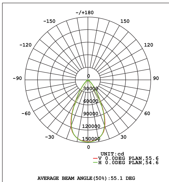
配光曲線
