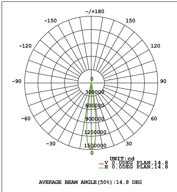
配光曲線
