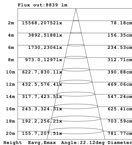
照度図
