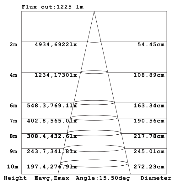
照度図
