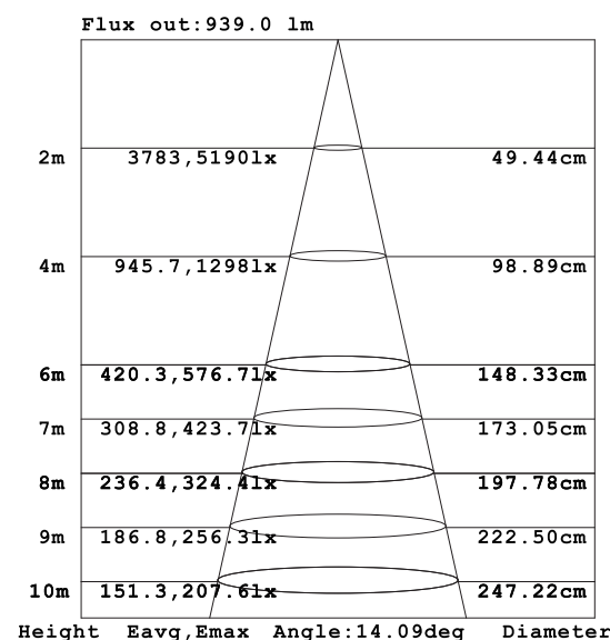
照度図
