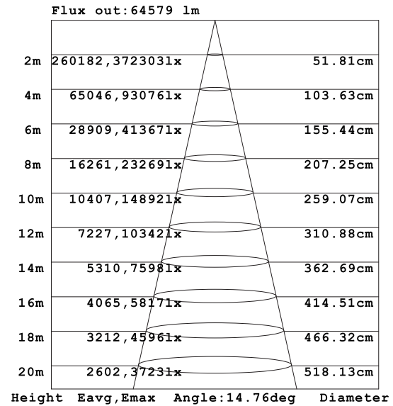
照度図
