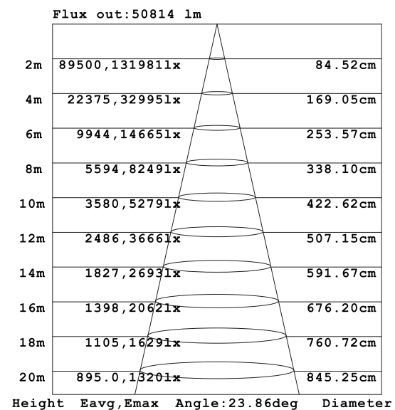
照度図
