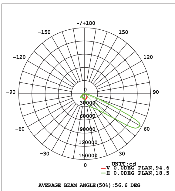
配光曲線
