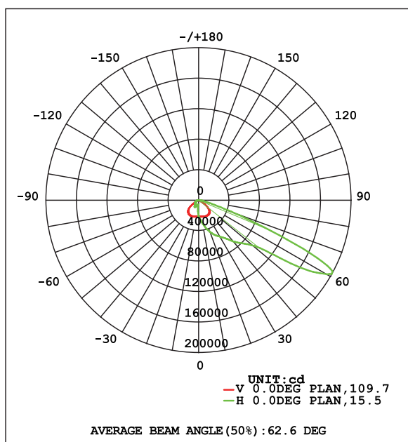
配光曲線
