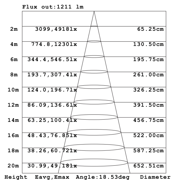
照度図
