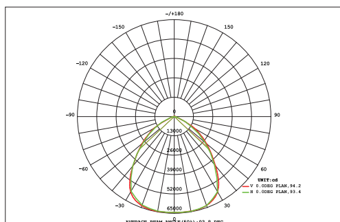
配光曲線
