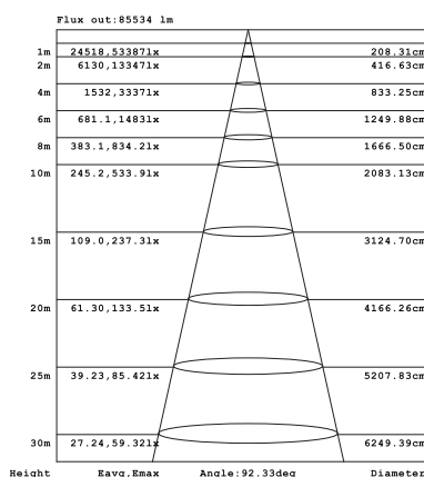
照度図
