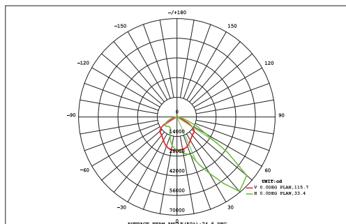
配光曲線
