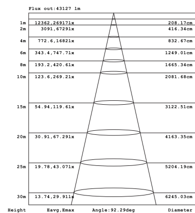
照度図
