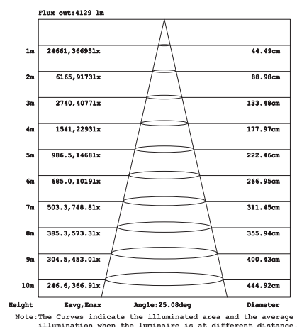
照度図
