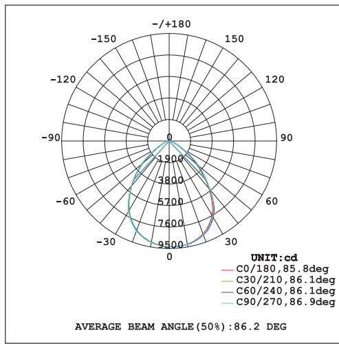
配光曲線
