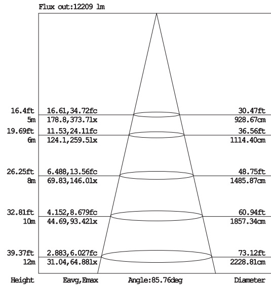
照度図
