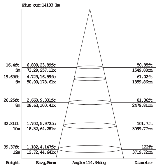
照度図
