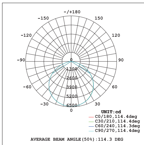
配光曲線
