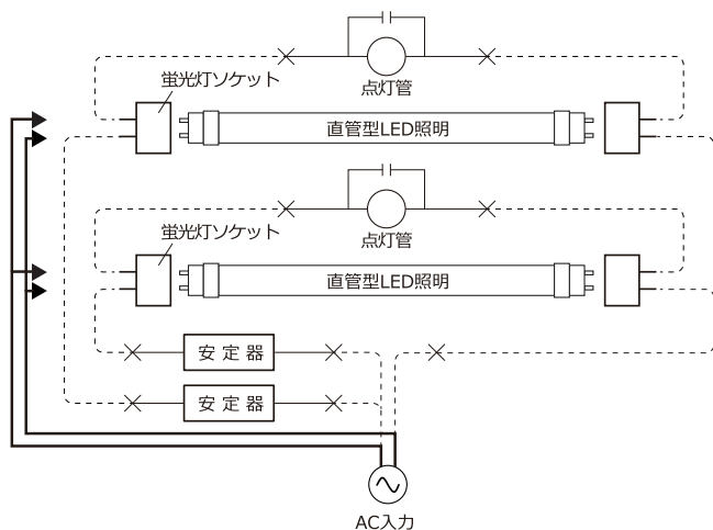
2灯用器具 結線例①
